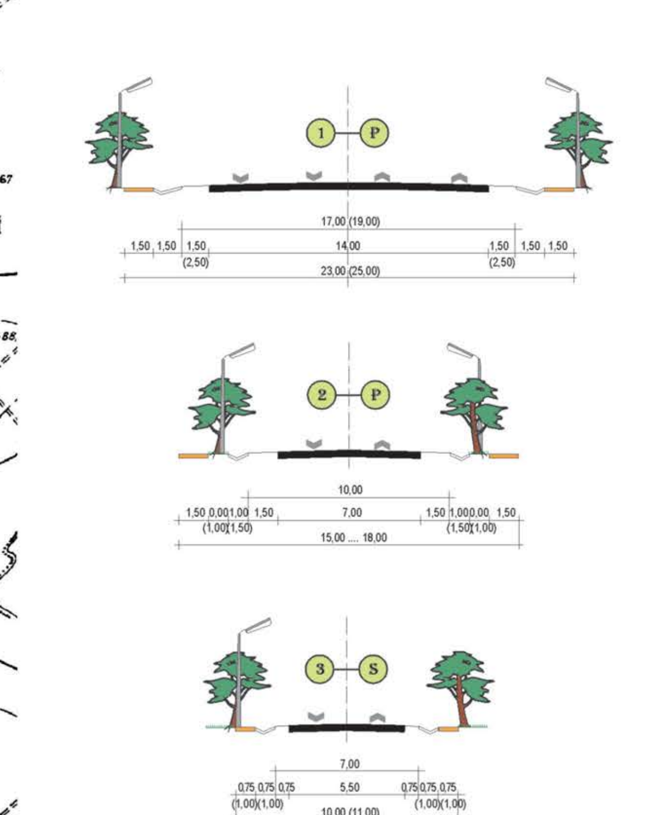
PROFILURI TRANSVERSALE CARACTERISTICE Sc. 1 / 200
